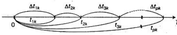
Рис. 5.1. Временная эпюра случайной ситуации при k -м опыте в случае мгновенного восстановления отказавшей системы путем замены элемента
